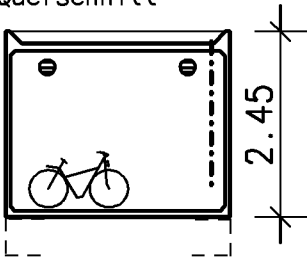
Querschnitt
