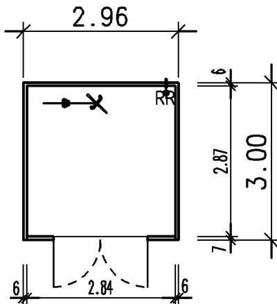
Grundriß
