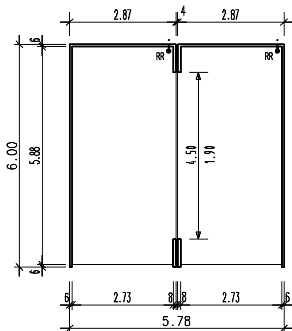
Grundriss
