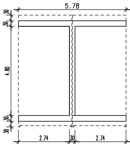
Gründung gem. Typenstatik
