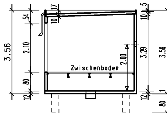
Längsschnitt
