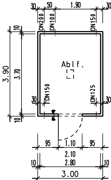
Grundriss
