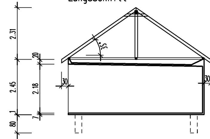
Längsschnitt
